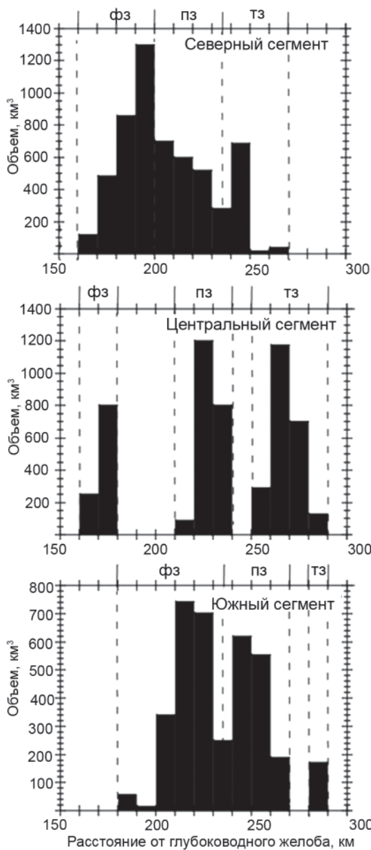
Рис. 4. Диаграммы зависимости суммарных объемов вулканитов от расстояний до глубоководного желоба.
